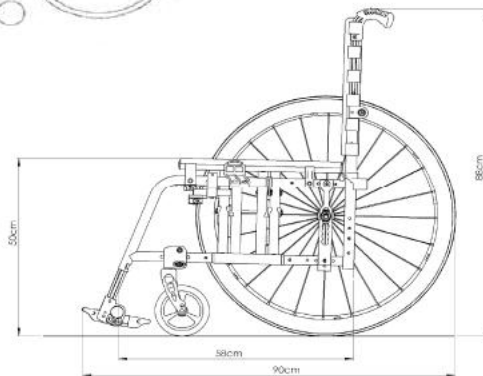
Abbildung: Stuhl mit ST 40 cm und 24" Rad
